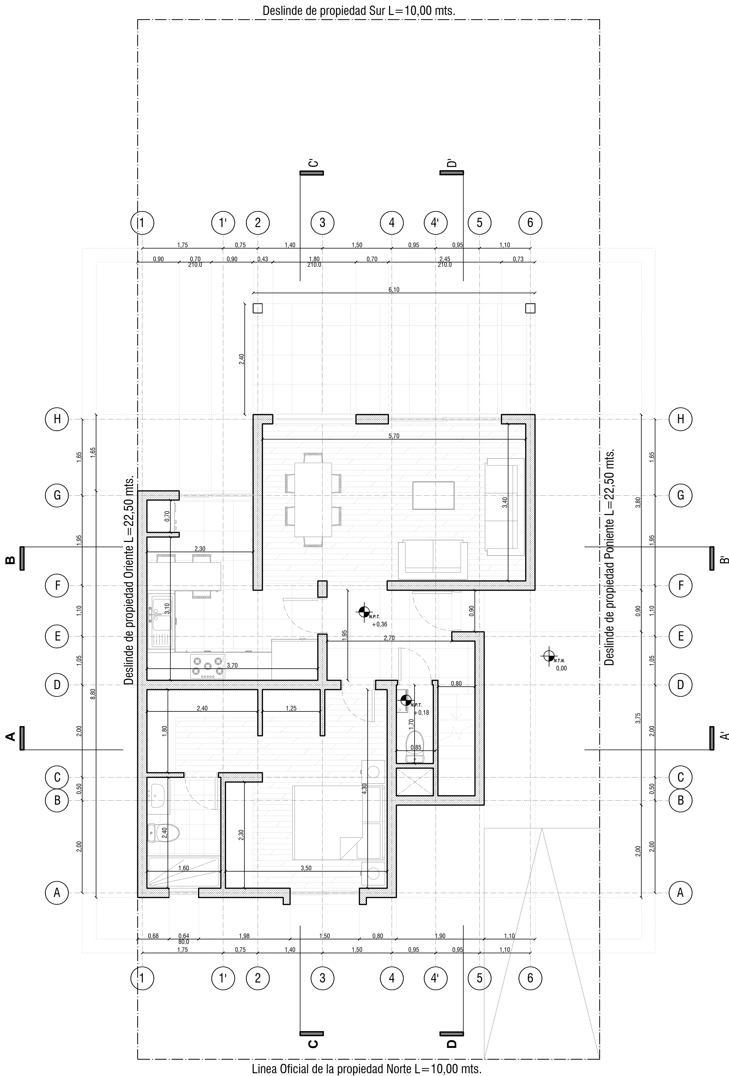
Planta Arquitectura Nivel 01 esc 1:50
