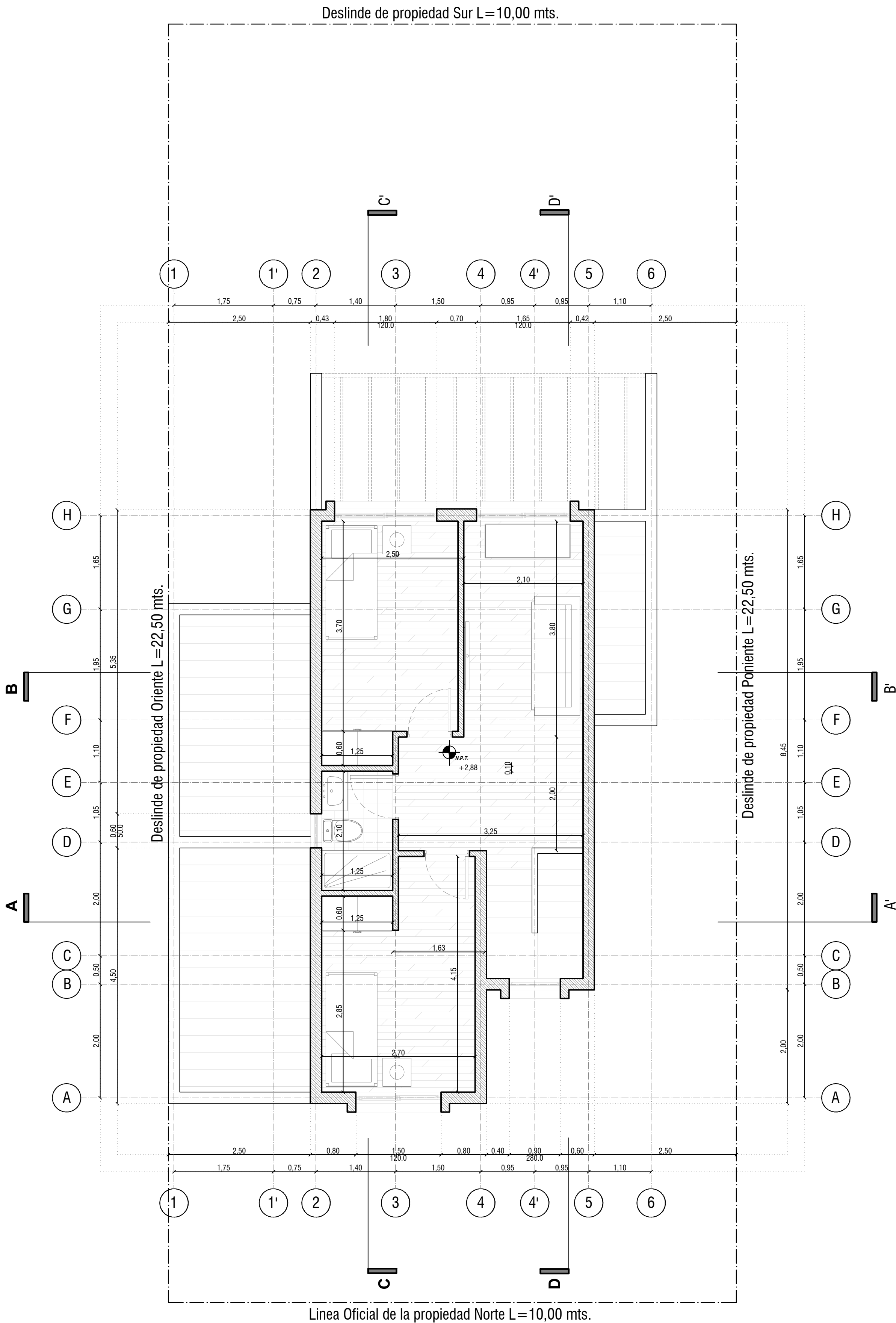
Planta Arquitectura Nivel 02 esc 1:50
